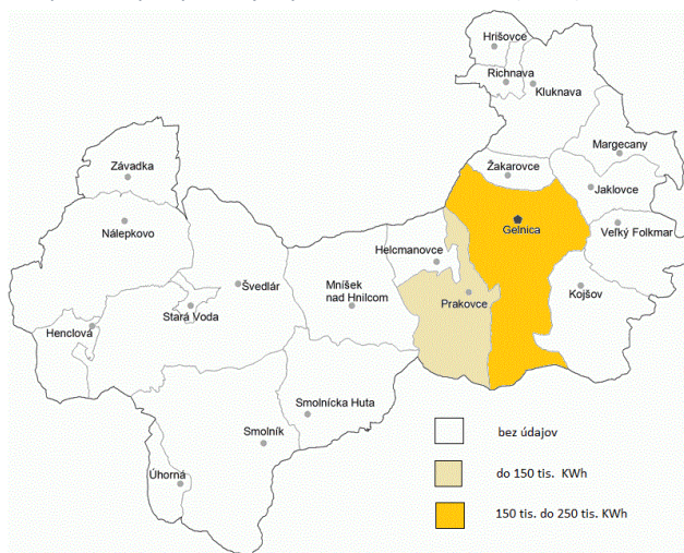
Mapa 6 Mapa spotreby tepla v okrese Gelnica. (2020).
