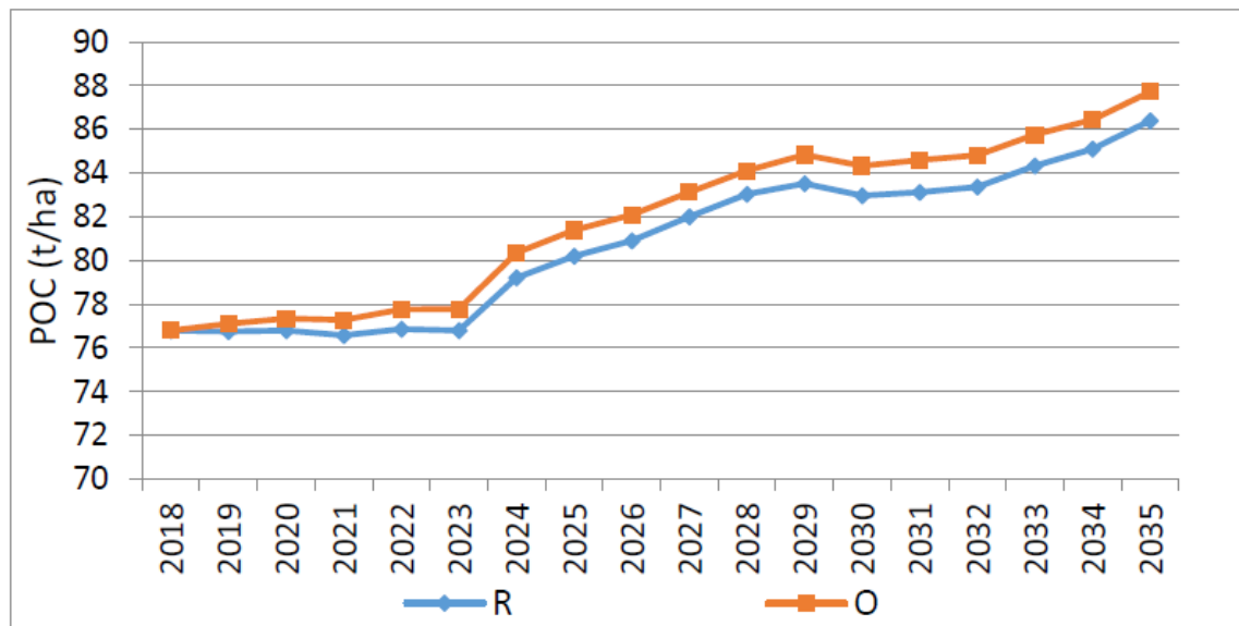
Graf 21 Porovnanie priemerných modelovaných zásob POC v horskom regióne pri aplikácii reálneho (R) a optimálneho (O) manažérskeho scenára
