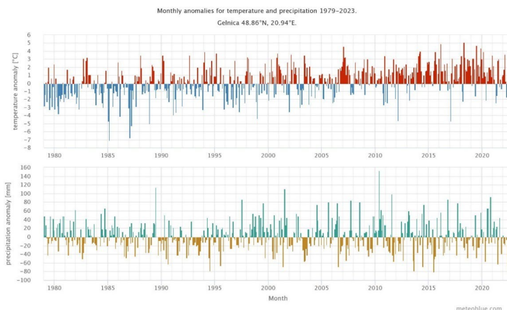
Graf 17 Graf mesačných anomálii teploty a zrážok v oblasti Gelnica v období rokov 1979-2021.
