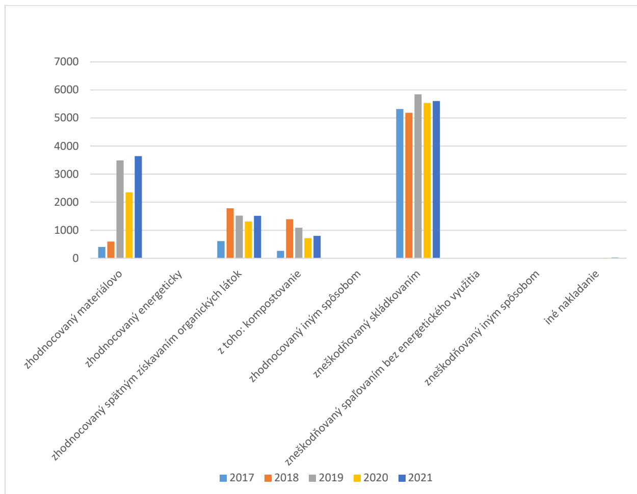
Graf 25 Množstvo komunálneho odpadu podľa spôsobu nakladania v okrese Gelnica v rokoch 2017 - 2021 (v tonách)
