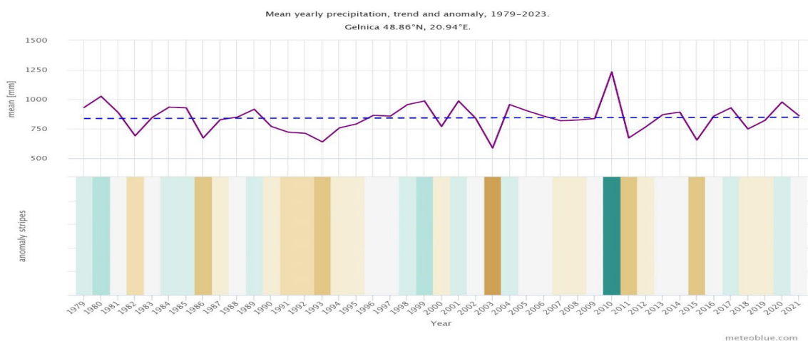
Graf 16 Ročný úhrn zrážok za obdobie rokov 1979-2021.
