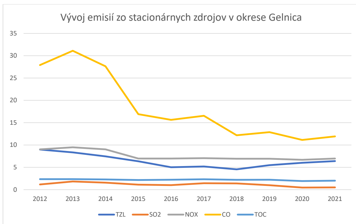
Graf 22 Vývoj emisií zo stacionárnych zdrojov (veľké a stredné zdroje znečistenia) v okrese Gelnica v období 2012-2021.
