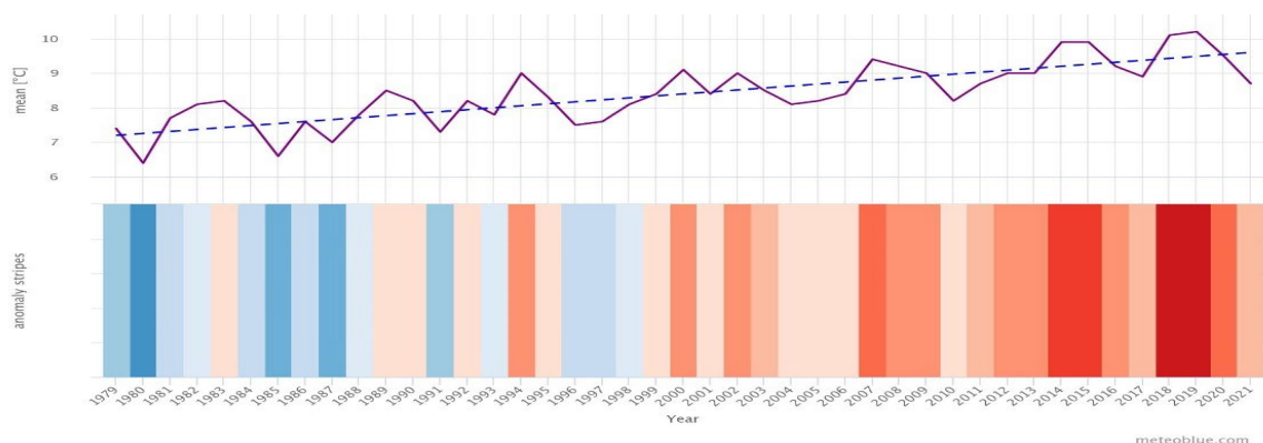
Graf 15 Priemerné ročné teploty v oblasti Gelnica v období 1979-2021.
